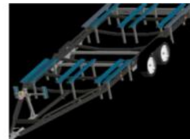
ALFA-T Marine 48125HP200P Pontoon szállító
